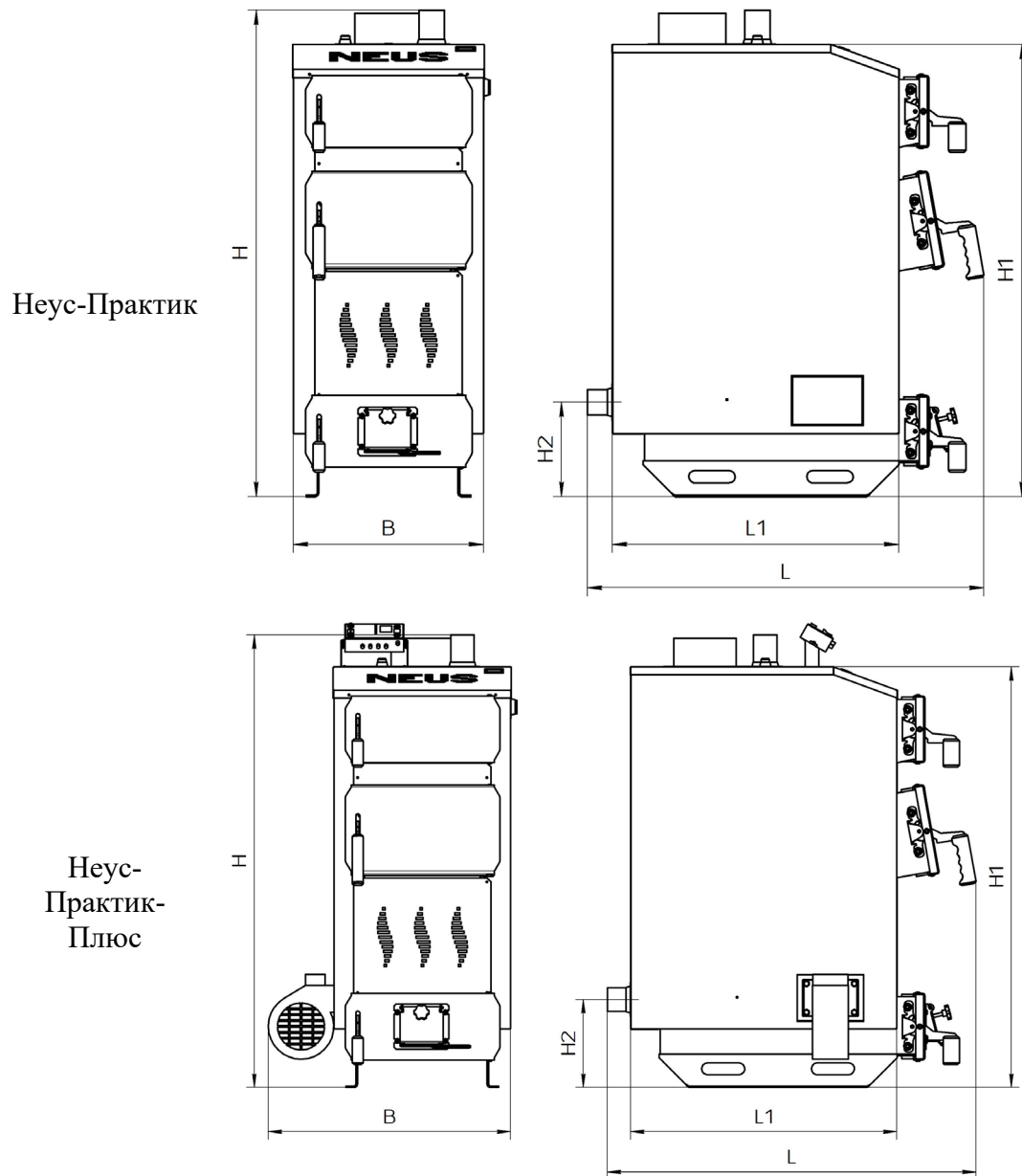
Рисунок 1 – Габаритне креслення котла Неус-Практик (Неус-Практик-Плюс)
