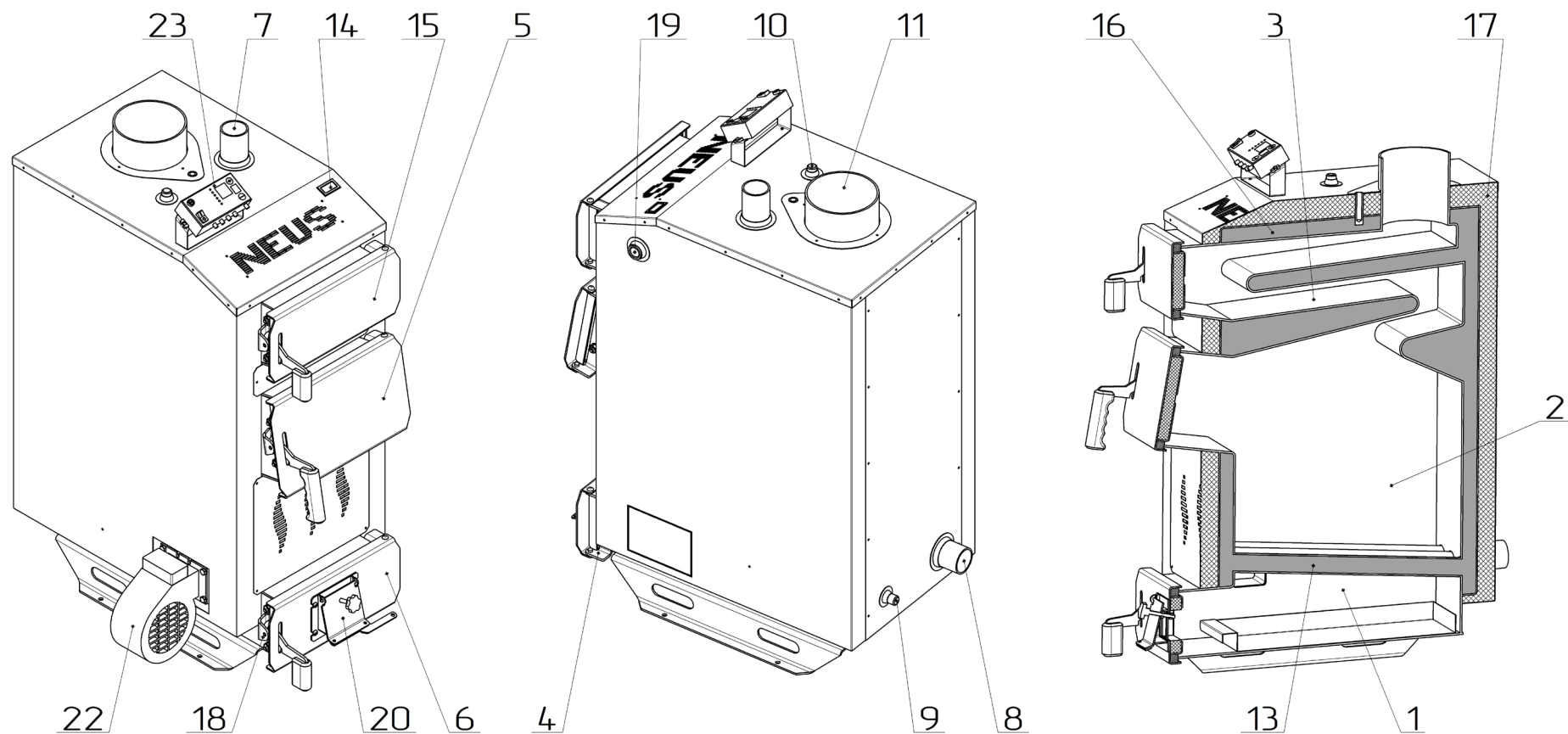
Рисунок 2б – Основні елементи котла Неус-Практик-Плюс
