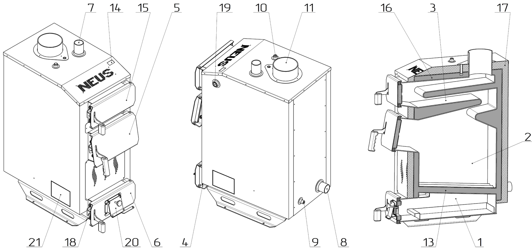
Рисунок 2а – Основні елементи котла Неус-Практик
