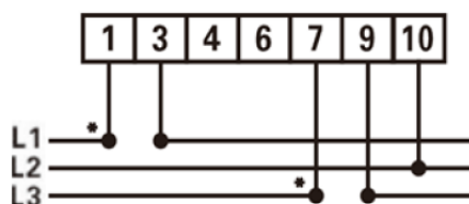
Рисунок 11. Трьохфазний трипровідний прилад: пряме підключення
