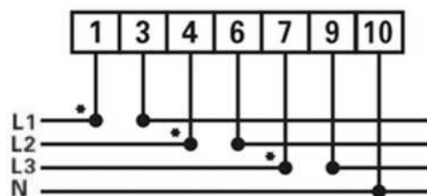
Рисунок 10. Трьохфазний чотирипровідний прилад: пряме підключення
