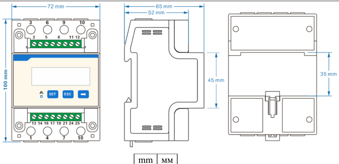
Рисунок 5. Схема розмірів контуру
