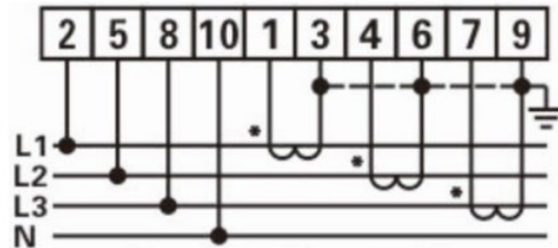
Рисунок 12. Трьохфазний чотирипровідний прилад: підключення через трансформатор струму
