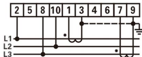
Рисунок 13. Трьохфазний трипровідний прилад: підключення через трансформатор струму
