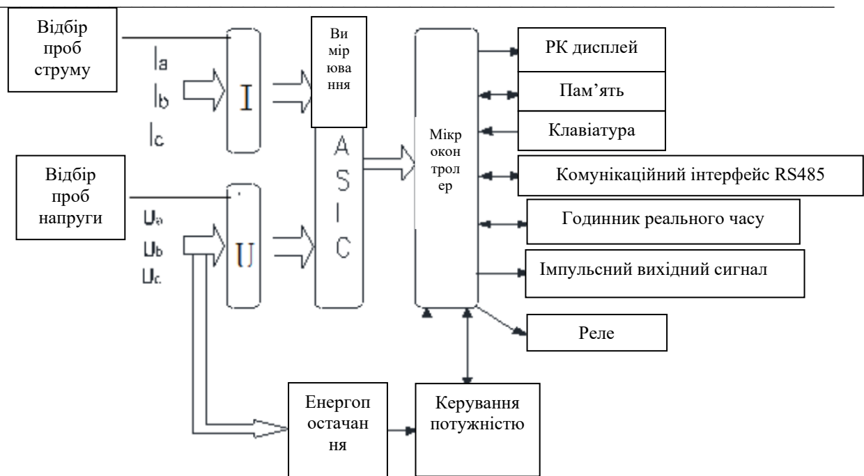
Рисунок 1. Блок-схема принципу роботи
