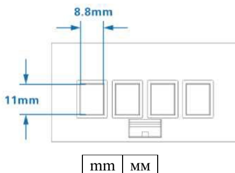
Рисунок 6. Клема кабелю струму (діапазон площі поперечного перерізу провідника \leq 16 \text{ mm}^2 )
