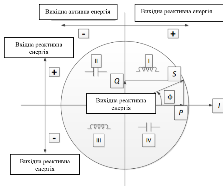
Рисунок 5. Принципова схема вимірювання енергії в чотирьох квадрантах
