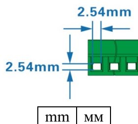
Рисунок 7. Клема кабелю RS485 (діапазон площі поперечного перерізу провідника 0,25\text{-}1 \text{ mm}^2 )
