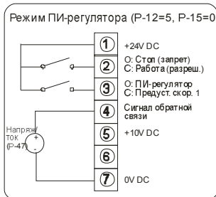
Режим ПИ-регулирования и предустановленная скорость 1
