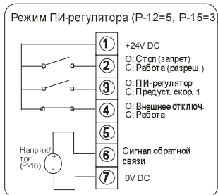
Режим ПИ-регулирования, предустановленная скорость 1 и термистор двигателя
