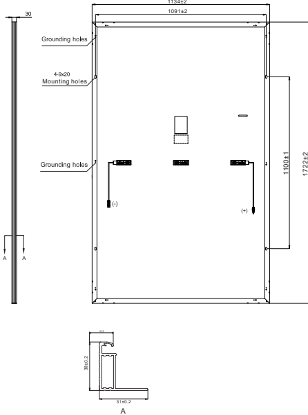
Розміри PV модуля, в мм
