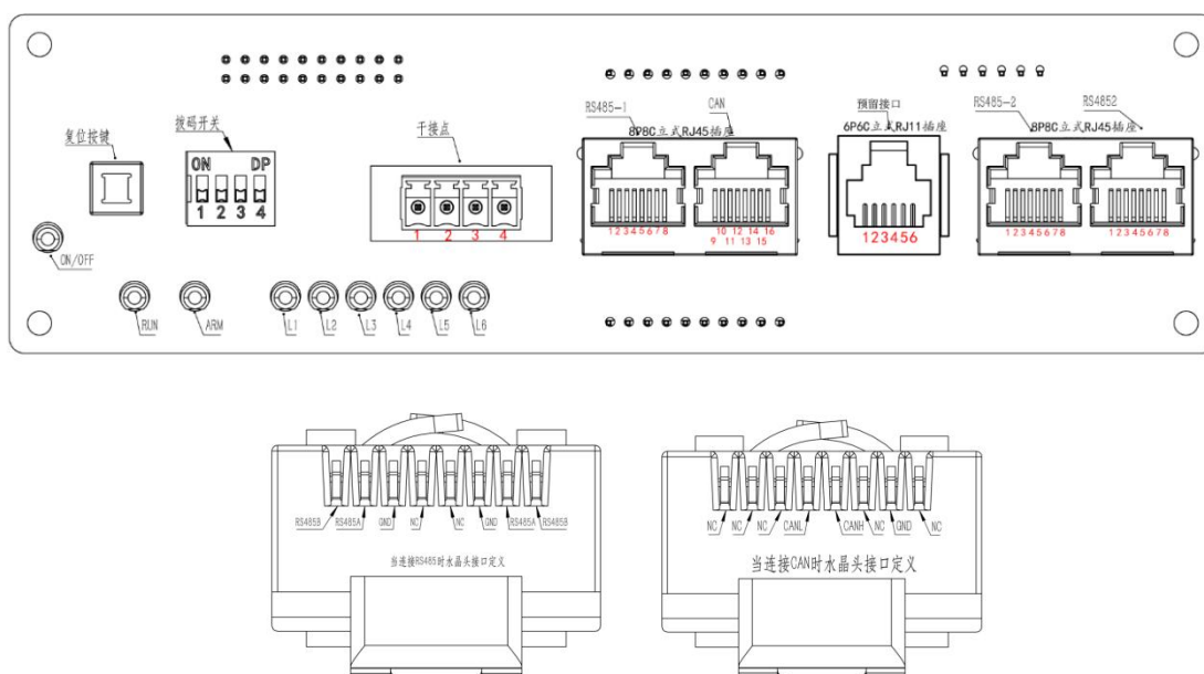
接口板接口示意图
