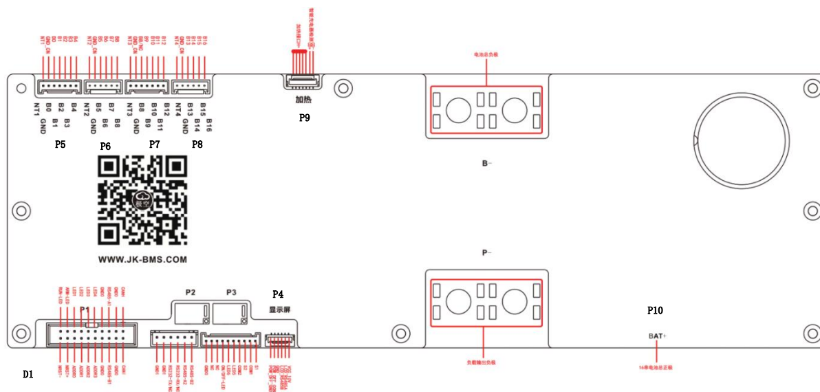
JK-PB1/2A16S-10/15/20P 连接器示意图
