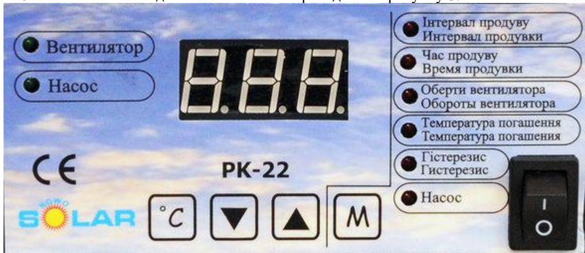
Рисунок 3 – Зовнішній вигляд передньої панелі контролера
