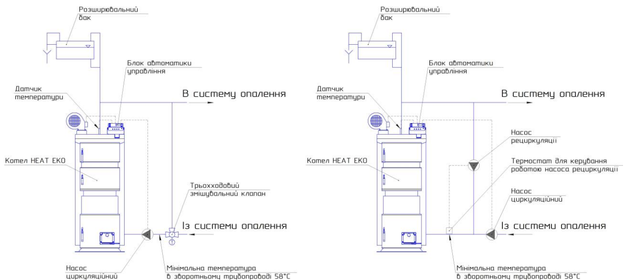
Рисунок 3 – Схема підключення котла до системи опалення
