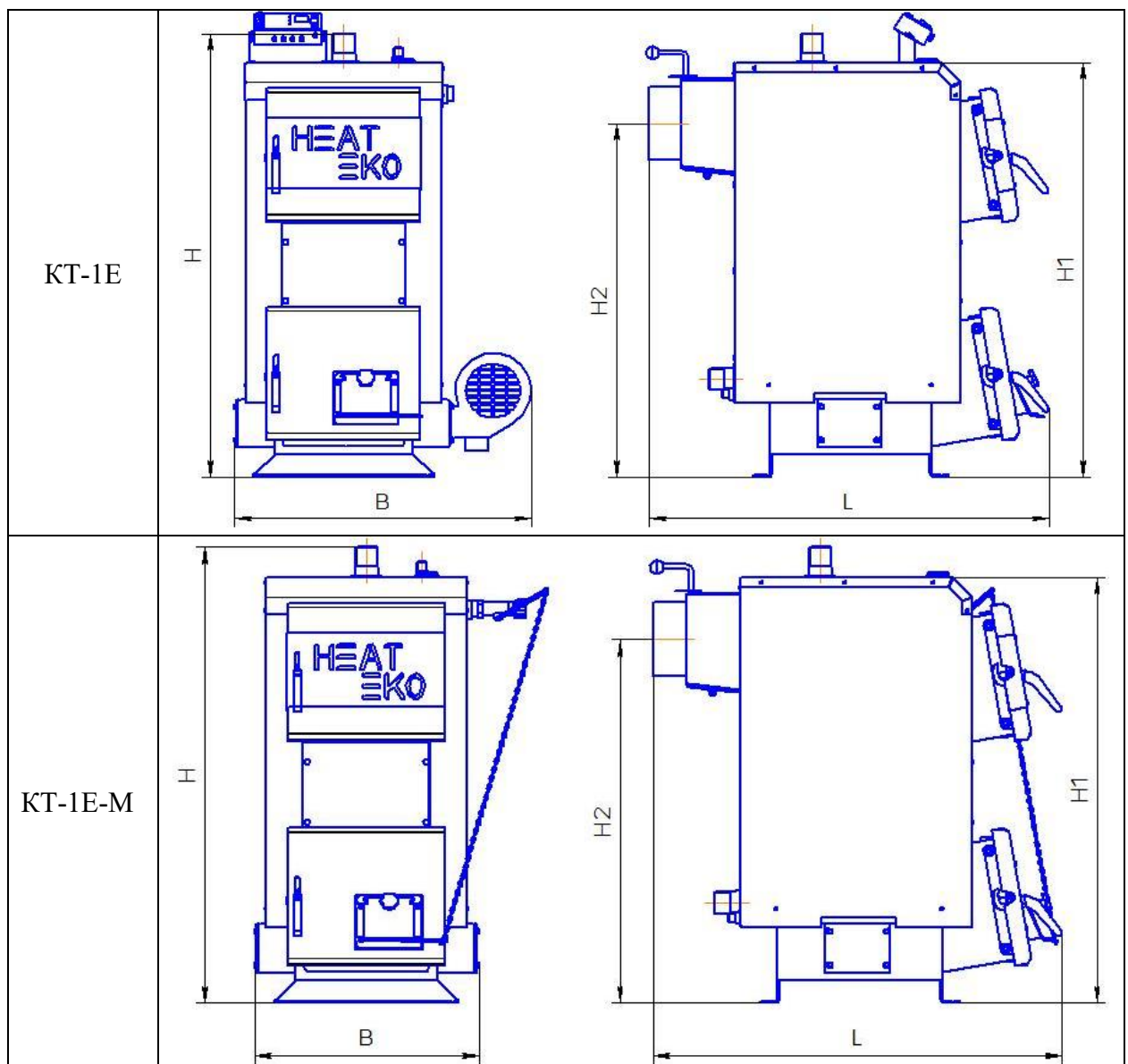
Рисунок 1 – Габаритне креслення котла КТ-1Е (КТ-1Е-М)
