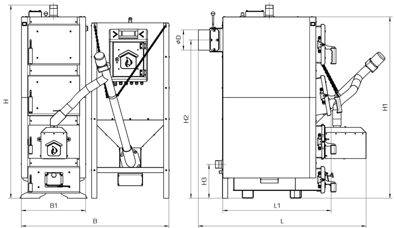
Рисунок 1 – Габаритне креслення котла
