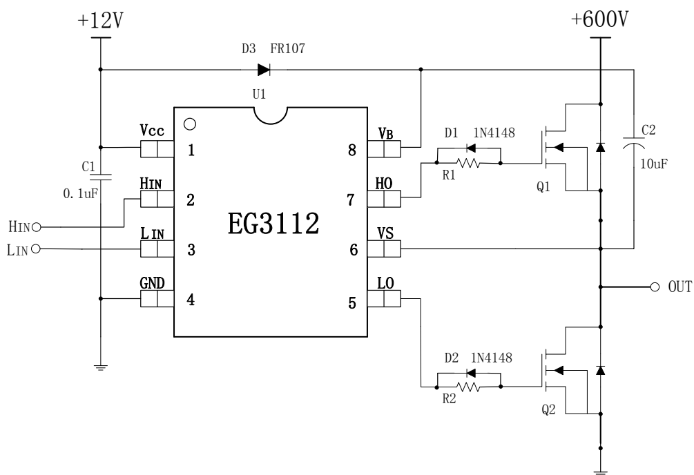
图 6-1. EG3112 典型应用电路图
