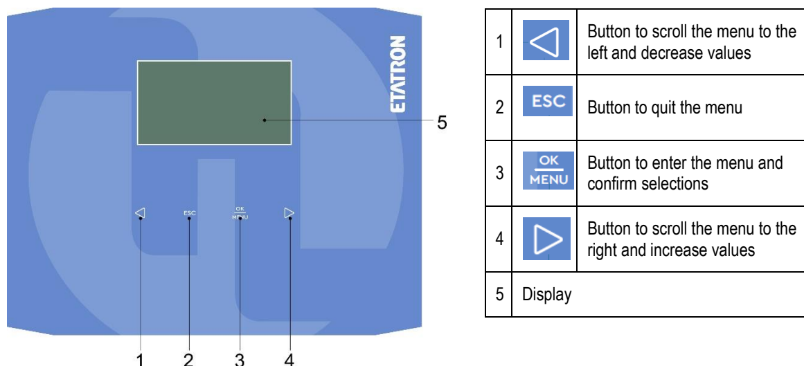
Fig. 4 – Keypad
