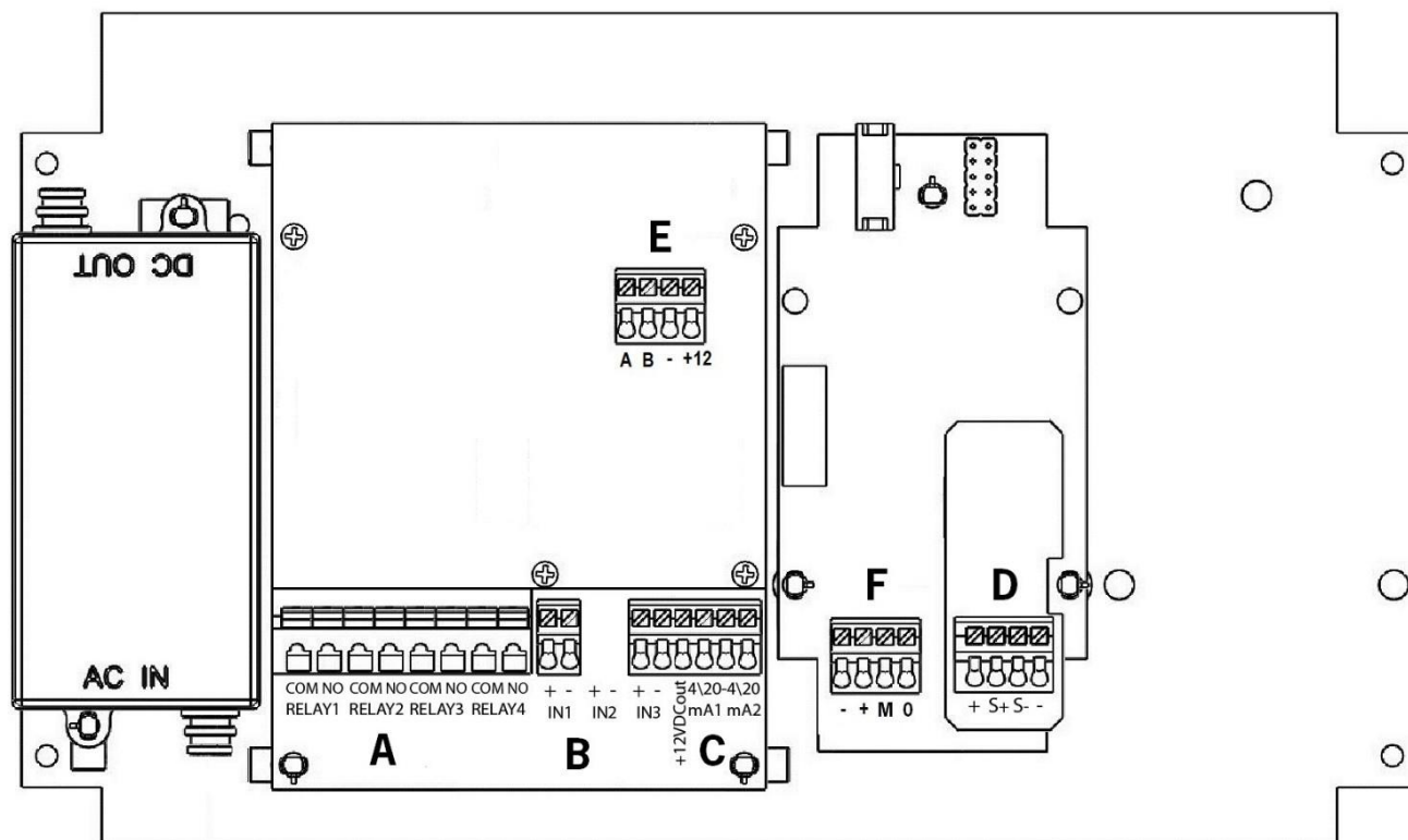
Fig. 3 – Schema di collegamento
