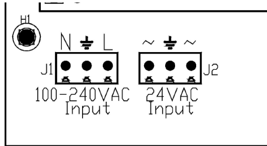
Fig. 1 – Collegamento elettrico
