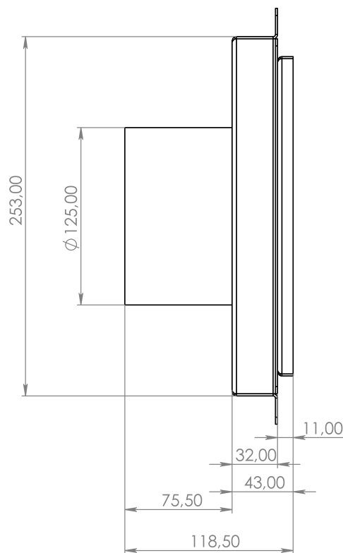
Вид збоку
