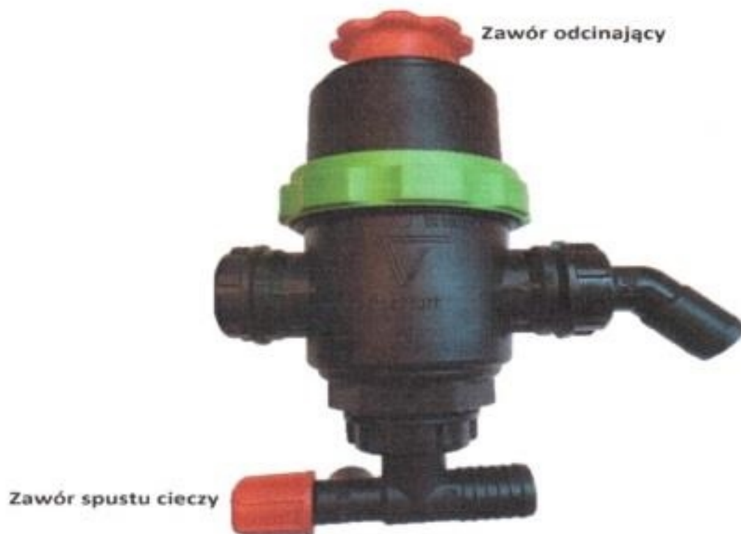
Rys.11.Filtr.
