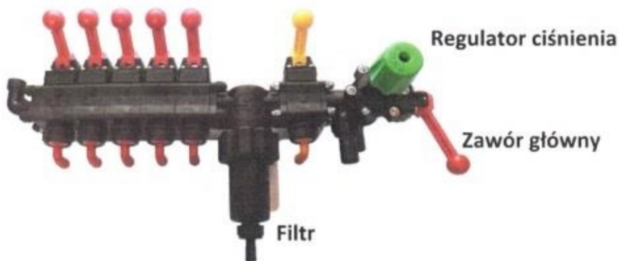
Rys.9. Budowa rozdzielacza.
