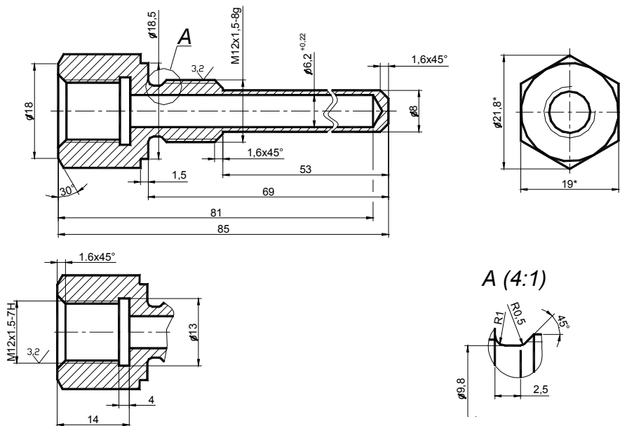
Рисунок Г.2 Гільза для датчика температури (з діаметром монтажної частини 6 мм і різьбою рухливого штуцера M12x1,5). Матеріал гільзи – прокат калібрований ГОСТ 1051, сталь 45 з покр. Ц6.хр, або 12Х18Н10Т (латунь не допускається)
