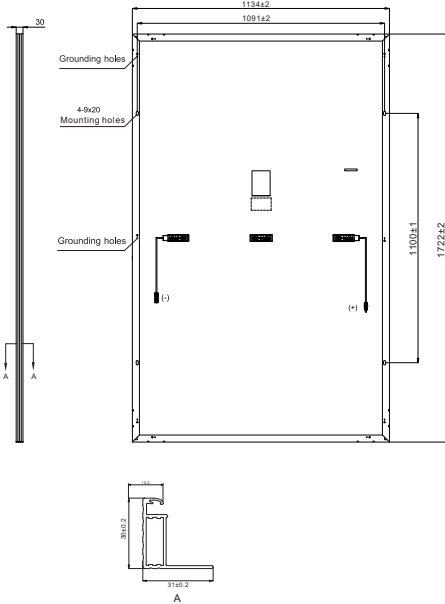
Розміри PV модуля, в мм
