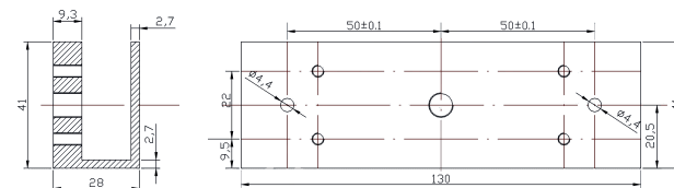
Кронштейн "UL"
