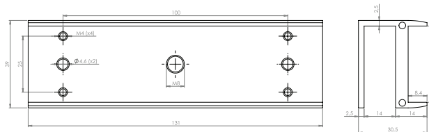
Кронштейн "U"
