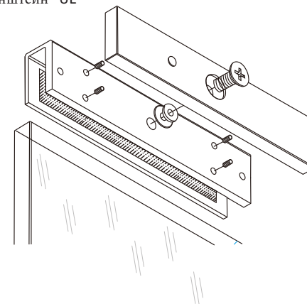
Кронштейн "UL"
