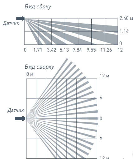
РИС. 3. Зона обнаружения датчика
