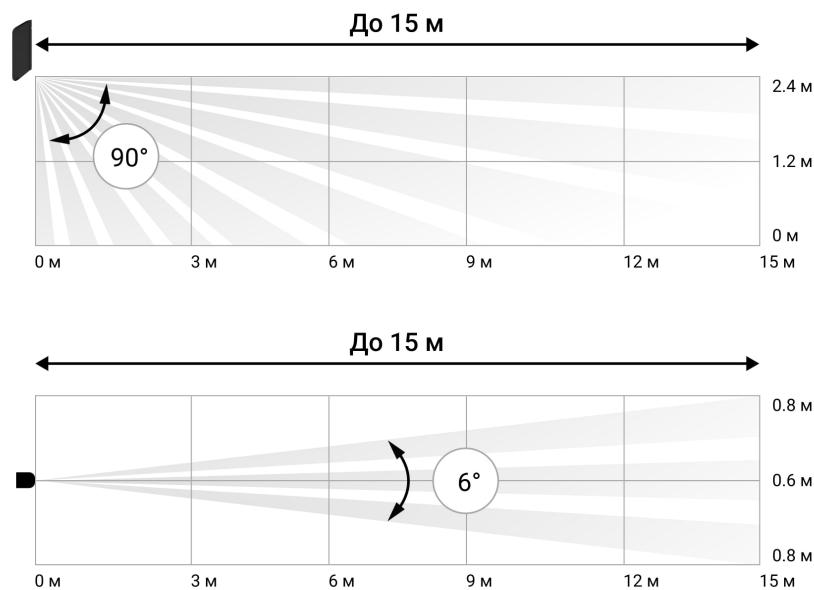
Горизонтальні та вертикальні кути огляду датчика
