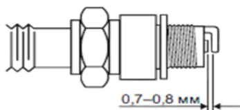
Рисунок 7. Величина зазору між електродами свічки запалювання.
