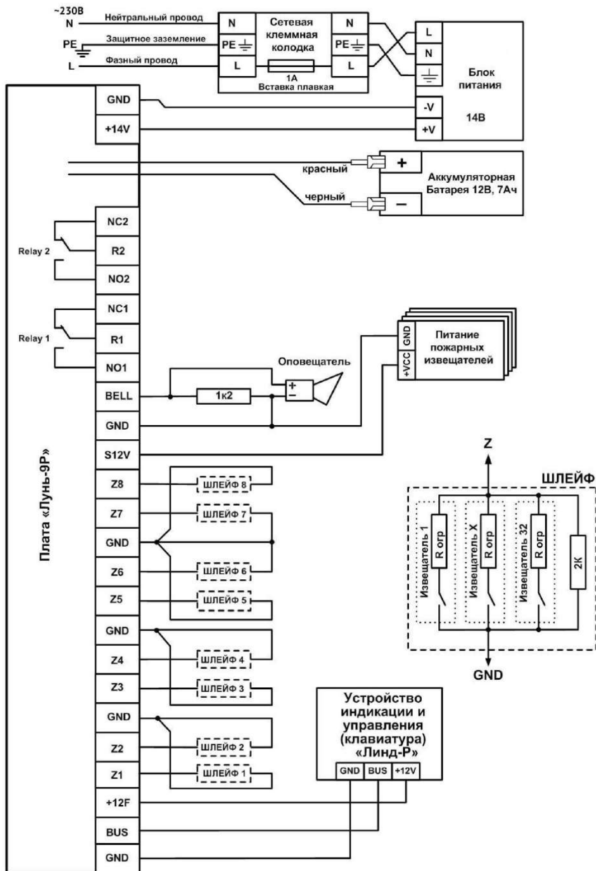
Рисунок 9. Схема подключения внешних устройств и извещателей
