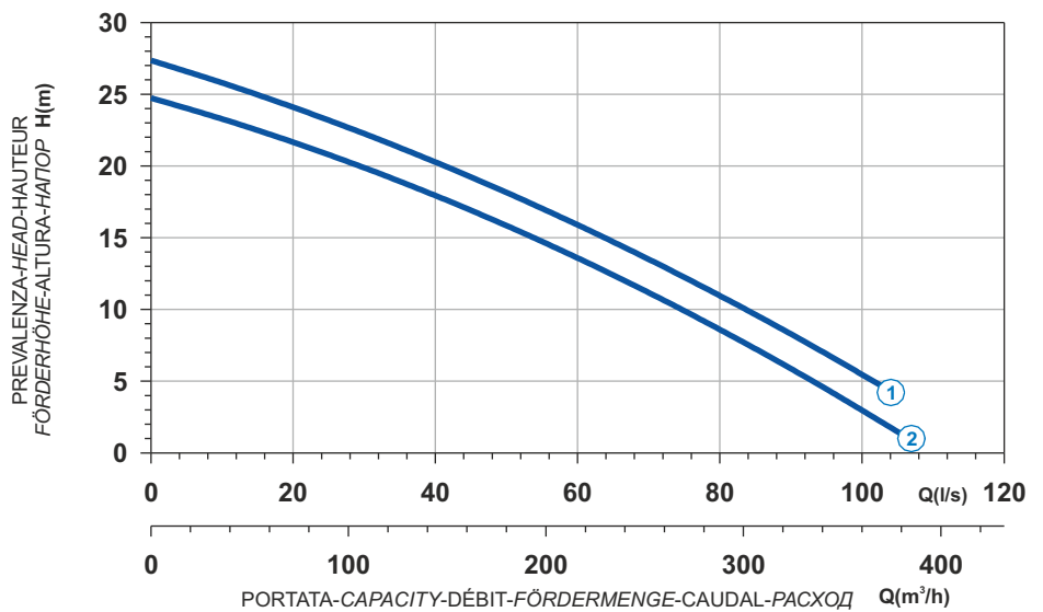
Curva caratteristica - Performance curve - Courbe caractéristique Kennlinie - Curva característica - Характеристическая кривая
