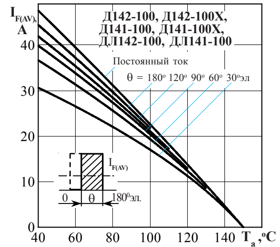
Рисунок 5 - Зависимость допустимого среднего прямого тока I_{F(AV)} от температуры окружающей среды T_a при естественном охлаждении на типовом охладителе при различных углах проводимости и для токов прямоугольной формы частотой f = 50 Гц и постоянного тока
