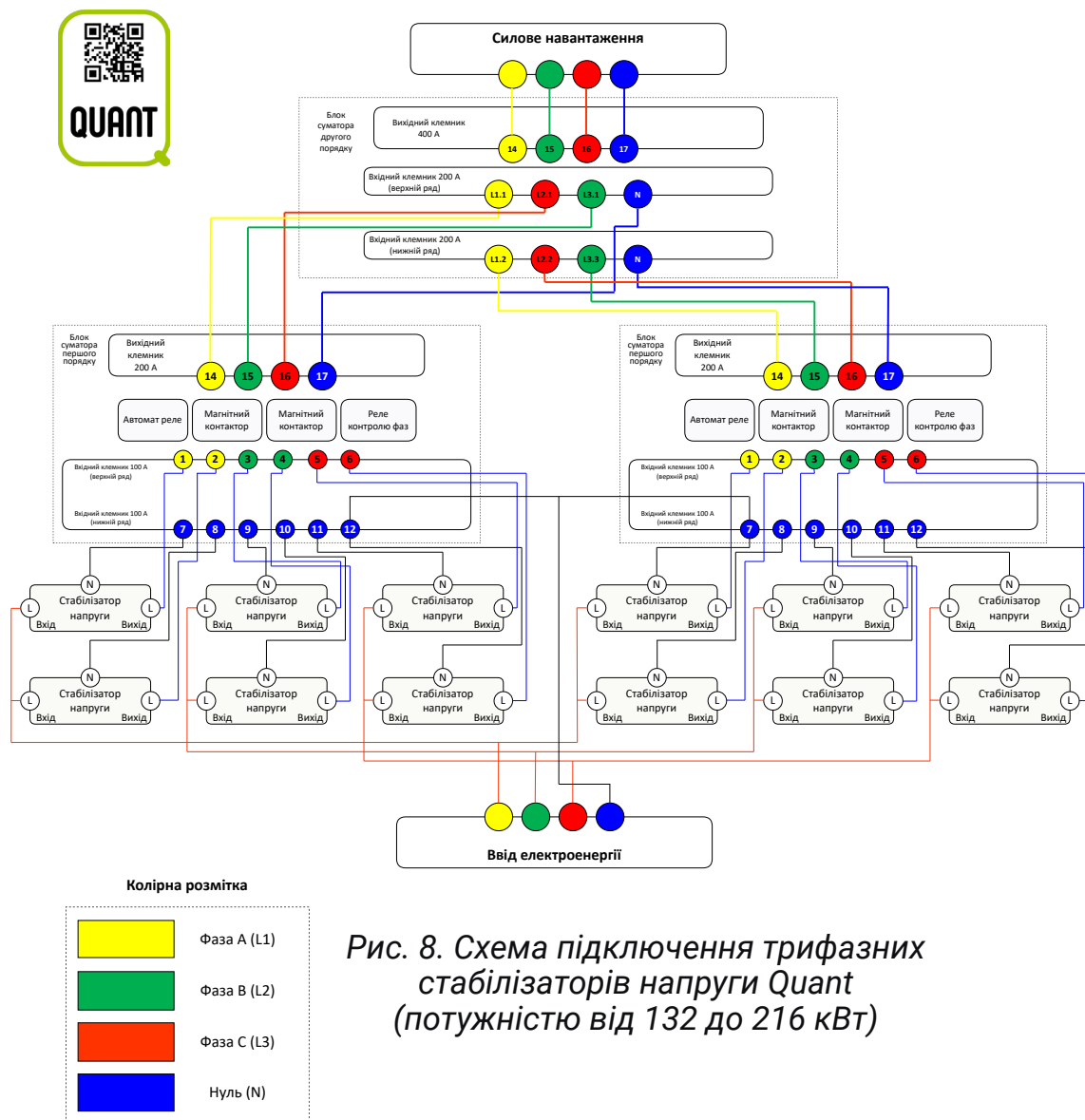
Загальна схема підключення трифазних стабілізаторів напруги Quant (потужністю від 132 до 216 кВт)
