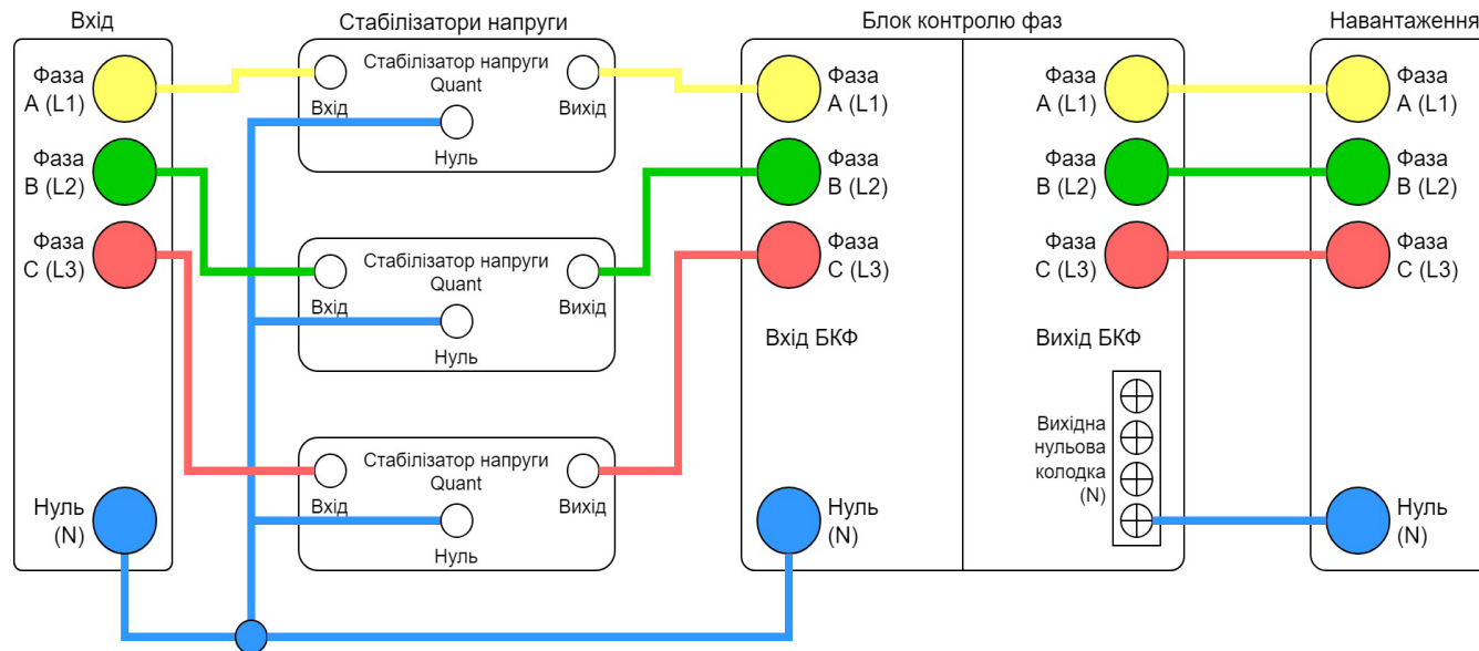
Рис. 4. Схема монтажу блоку контролю фаз
