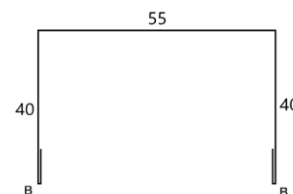
П-планка бокова
