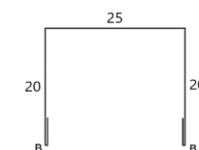
П-планка бокова
