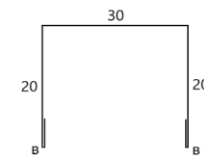
П-планка накривна
