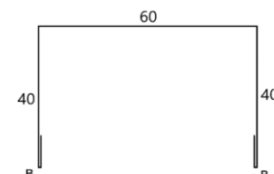
П-планка накривна
