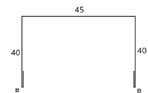
П-планка накривна
