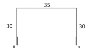
П-планка бокова
