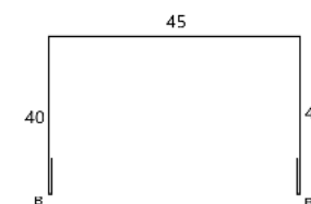
П-планка накривна
