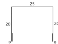
П-планка бокова
