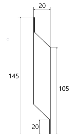
П-планка бокова
