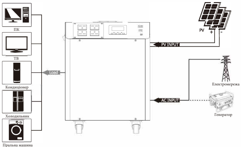
Рисунок 1: гібридна система виробництва електроенергії
