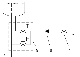
Fig. 4: Sistemul deschis (nepresurizat)
