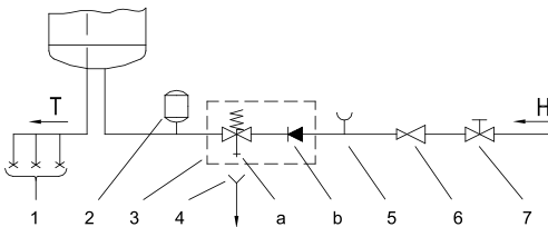
Малюнок 3: Напірна (закрита) система
