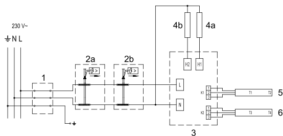
Рисунок 6: Электросхема
