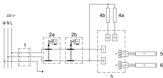
Fig. 6: Instalația electrică
