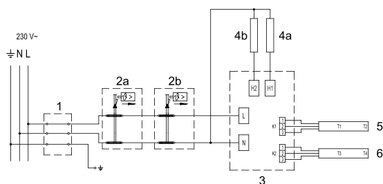
Мал. 6: Електросхема
