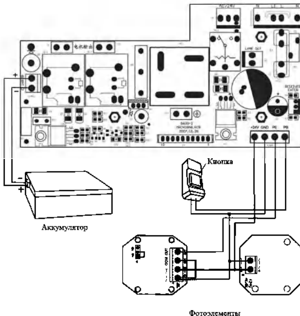
Рис. 4. Электрические подключения
