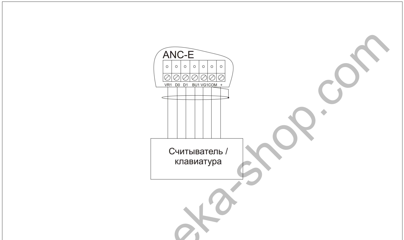
Рис.3. Подключение считывателя по интерфейсу Weigand.
