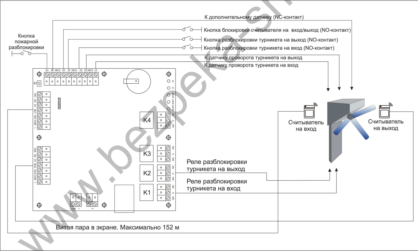
Рис 7.Функциональная схема оборудования точки прохода на основе турникета с независимым получением информации о факте прохода по входу и выходу. Вариант. Подключение питания, связи с управляющим контроллером и считывателей по интерфейсу Wiegand производится согласно пунктов 7.1-7.4 . Функциональное назначение информационных шлейфов и контактов реле указано в таблицах ниже.
