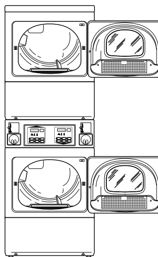
вид спереди
