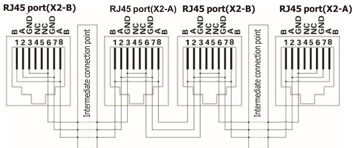
Схема з'єднання паралельних кабелів RS485
