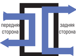
Конструкция «двойное U» Присоединения на задней стороне для компоновки Схема потоков – «двойное U»
