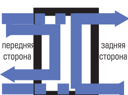
Конструкция «Двойное U плюс F3/F4» Предпочтительное исполнение для тепловых насосов с гнездами для датчиков Схема потоков – «Двойное U»
