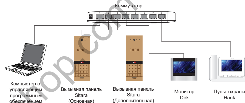
Схема 2. Пример подключения панели Sitara к локальной сети.
