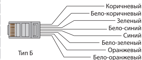
Обжим сетевого разъема RJ-45
