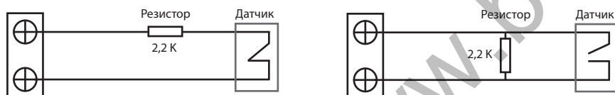
Подключение для нормально закрытых контактов Подключение для нормально открытых контактов
