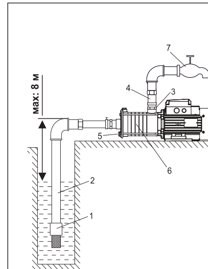
Коректний монтаж
