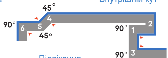
Підвіконня
