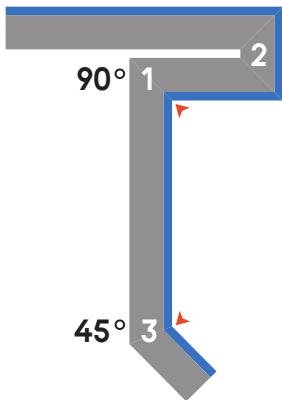
Відлив
