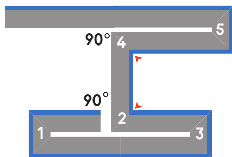
Виносний Карниз
