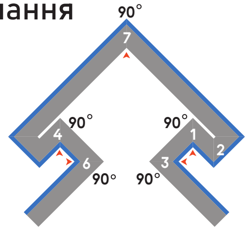
Зовнішній Кут
