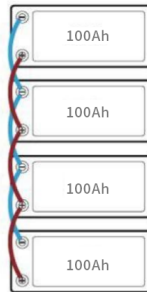
Паралельне підключення 24В(25,6В) 400Ah
