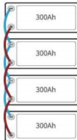
Паралельне підключення 12B(12,8V) 1200Ah
