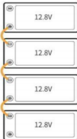
Послідовне підключення 48V(51,2V) 300Ah
