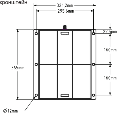
Настінний кронштейн
