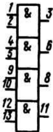
Условное графическое обозначение К533ЛИ2
