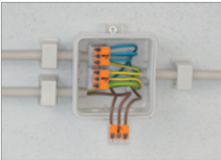
Электромонтаж тонких многожильных проводников в распределительной коробке.
