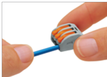
Затем опустите рычаг, чтобы замкнуть зажим.
