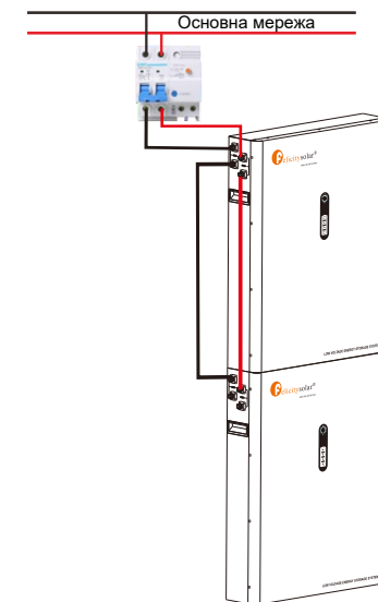
Крок 2: Схематичне зображення паралельного з'єднання двох акумуляторних блоків показано на рисунку 2.
