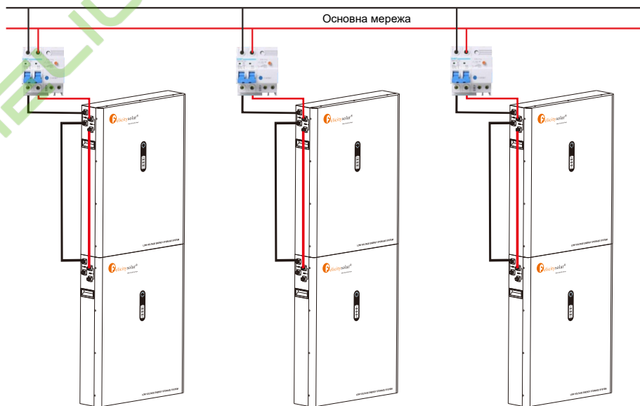
Крок 3: Схематичне зображення паралельного з'єднання шести акумуляторних блоків показано на рисунку 3.
