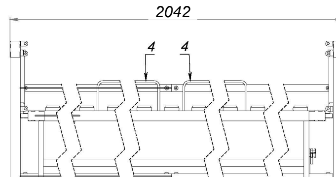
E-E (1 : 5)
