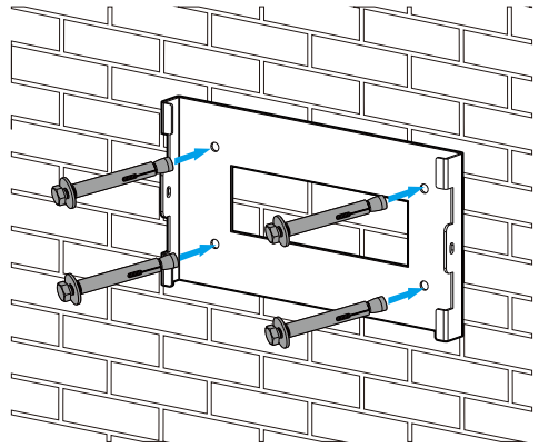
Рис. 4.5 Встановлення підвісної панелі інвертора
