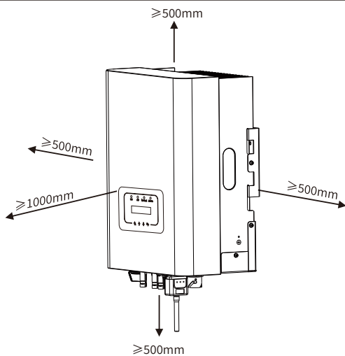
Рис. 4.3 Монтажний проміжок
