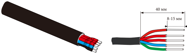
Рис. 5.8 Смугастий кабель змінного струму
