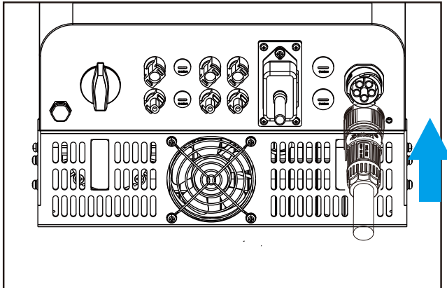
Рис. 5.10 Підключення входу змінного струму
