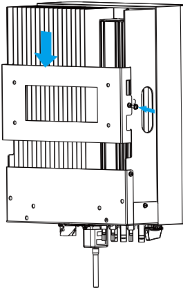
Рис. 4.6 Встановлення інвертора
