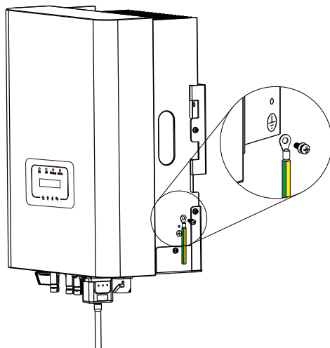
Рис. 5.11 Встановлення дроту заземлення оболонки
