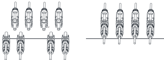
Рис. 5.6 Підключення входу постійного струму
