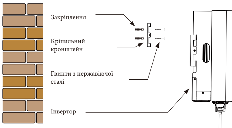
Рис. 4.4 Встановлення інвертора
