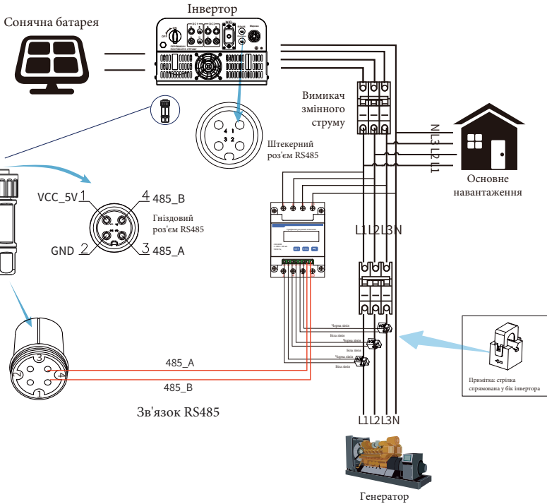
Рис. 7.14 Схема підключення лічильника CHNT
