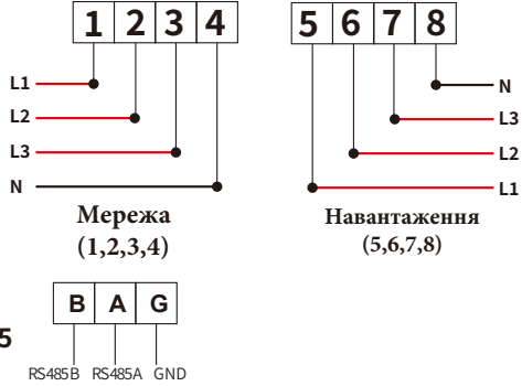
Рис. 7.18 Лічильник Eastron
