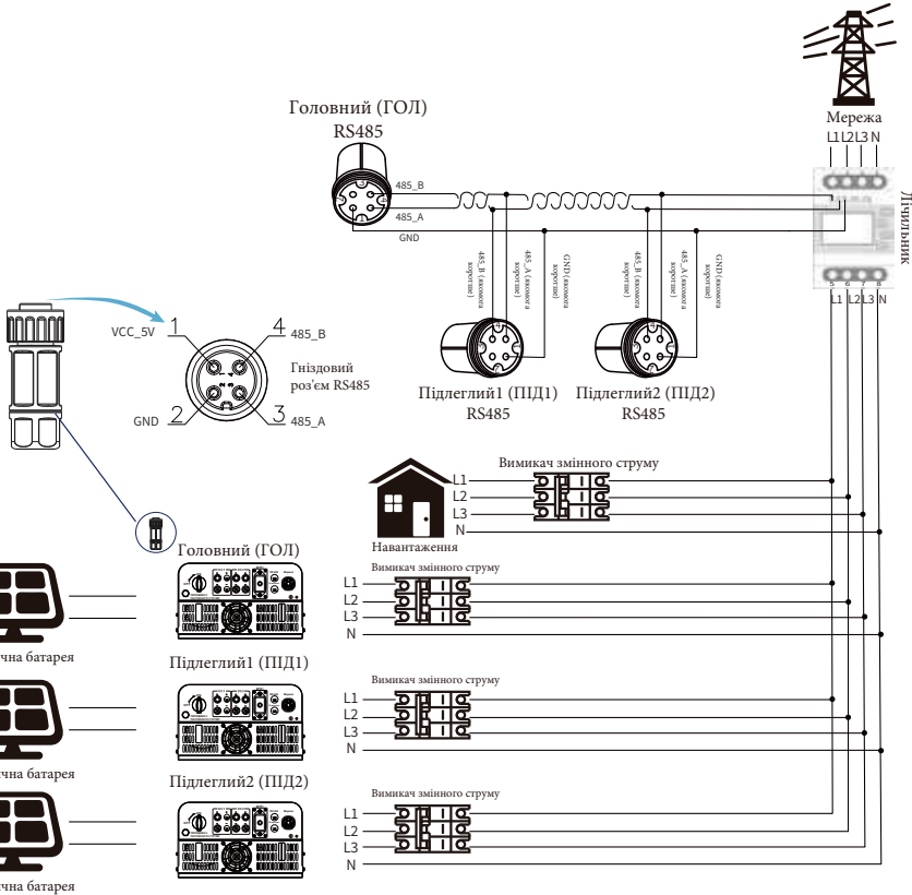
Рис. 7.19 Схема підключення Eastron (таблиця пропускнуної здатності)
