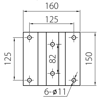
Розміри кронштейна
