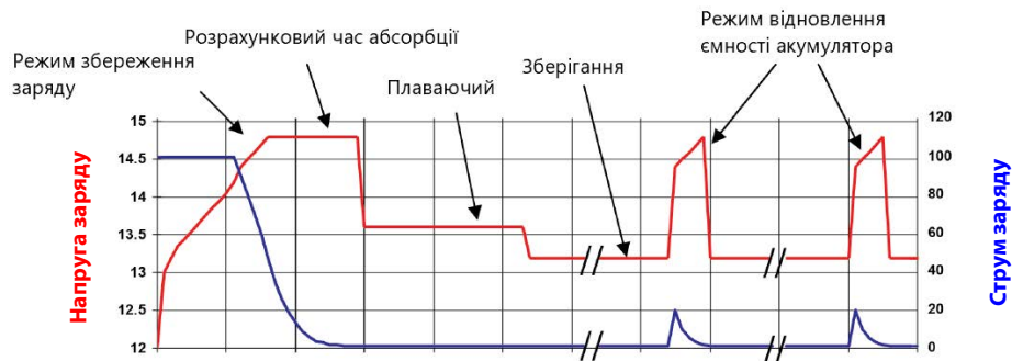
Мал. 4: Чотириступенева адаптивна крива заряду
