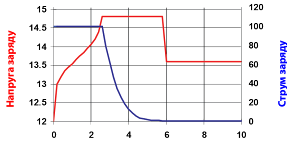
Мал. 3: Триступенева крива заряду
