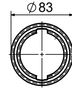
4-Dolum Boğazı (Filling Neck Ø60mm)
