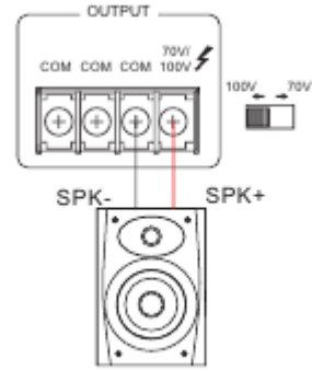
Мал. 5.2 Підключення гучномовців 100 В.
