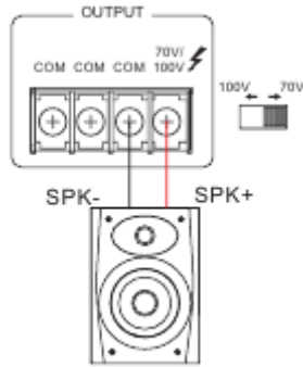
Мал. 5.1 Підключення гучномовців 70 В.
