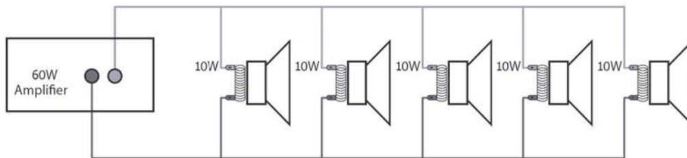
Мал. 5.3 Підключення трансформаторних гучномовців.
