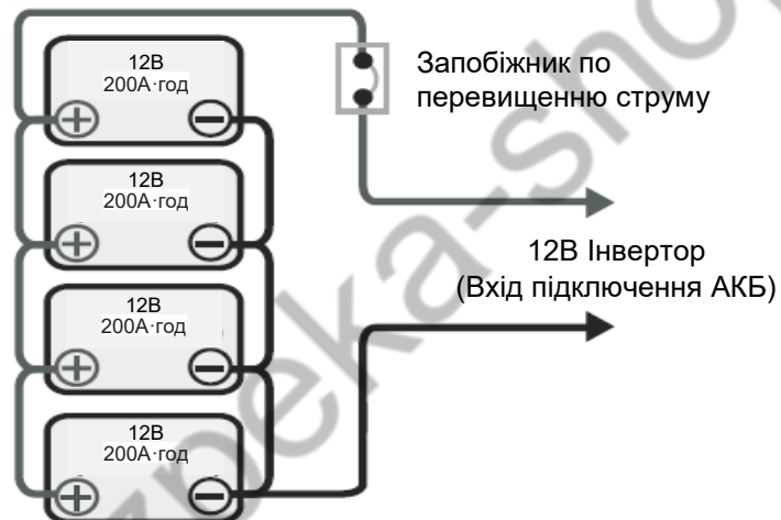
Рис. 6 Паралельне підключення батарей
