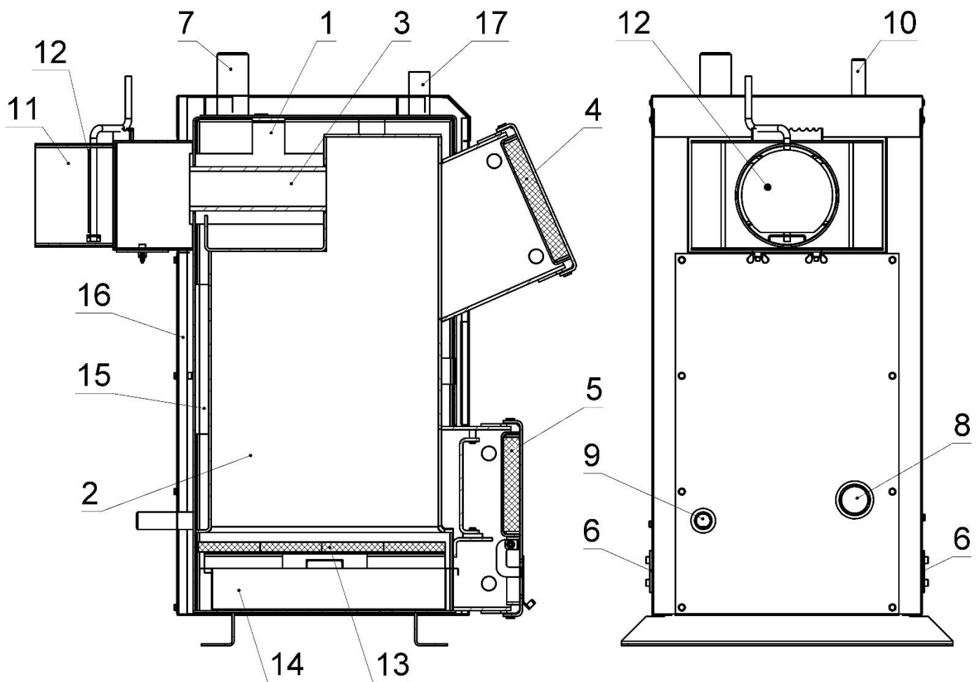
Рисунок 5.1 – Зовнішній вигляд та основні елементи котла
