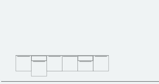
COMP. SA1399 L. 3168 x P. 490 x H. 880 mm
