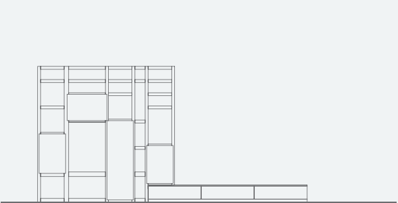
COMP. SA1376 L. 3580 x P. 362/490 x H. 1809 mm
