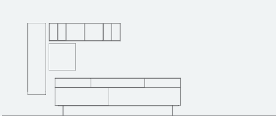
COMP. SA1505 L. 2474/3300 x P. 359/503 x H. 1950 mm
