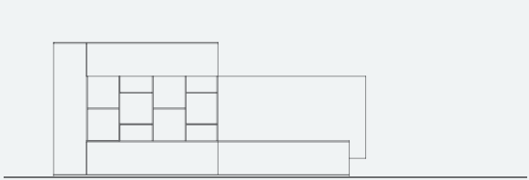
COMP. SA1501 L. 3344 x P. 361/490 x H. 1451 mm
