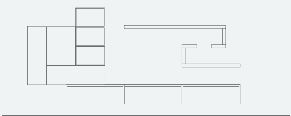
COMP. SA1384 L. 3872 x P. 361 x H. 1960 mm
