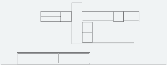
COMP. SA1506 L. 4048 x P. 359/487/490 x H. 2093 mm
