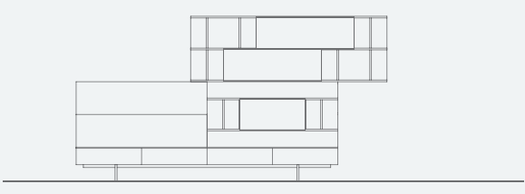
COMP. SA1504 L. 3344 x P. 352/490 x H. 1773 mm
