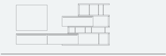
COMP. SA1508 L. 3168 x P. 250/361/490 x H. 1720 mm
