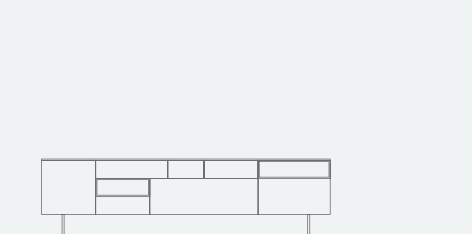
COMP. SA1400 L. 2816 x P. 503 x H. 778 mm
