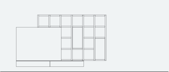
COMP. SA1396 L. 2816 x P. 362/423/490 x H. 1800 mm
