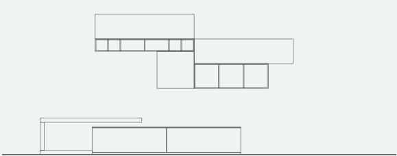
COMP. SA1503 L. 3600 x P. 250/359/490 x H. 2000 mm
