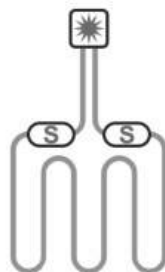
Схема укладки одножильного кабелю TXLP/1
